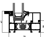
dwarsdoorsnede vaste raam
